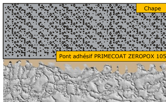
Pose de la chape dans les 15 minutes qui suivent l'application et la pénétration par massage du pont adhésif PRIMECOAT ZEROPOX 105 dans le support
